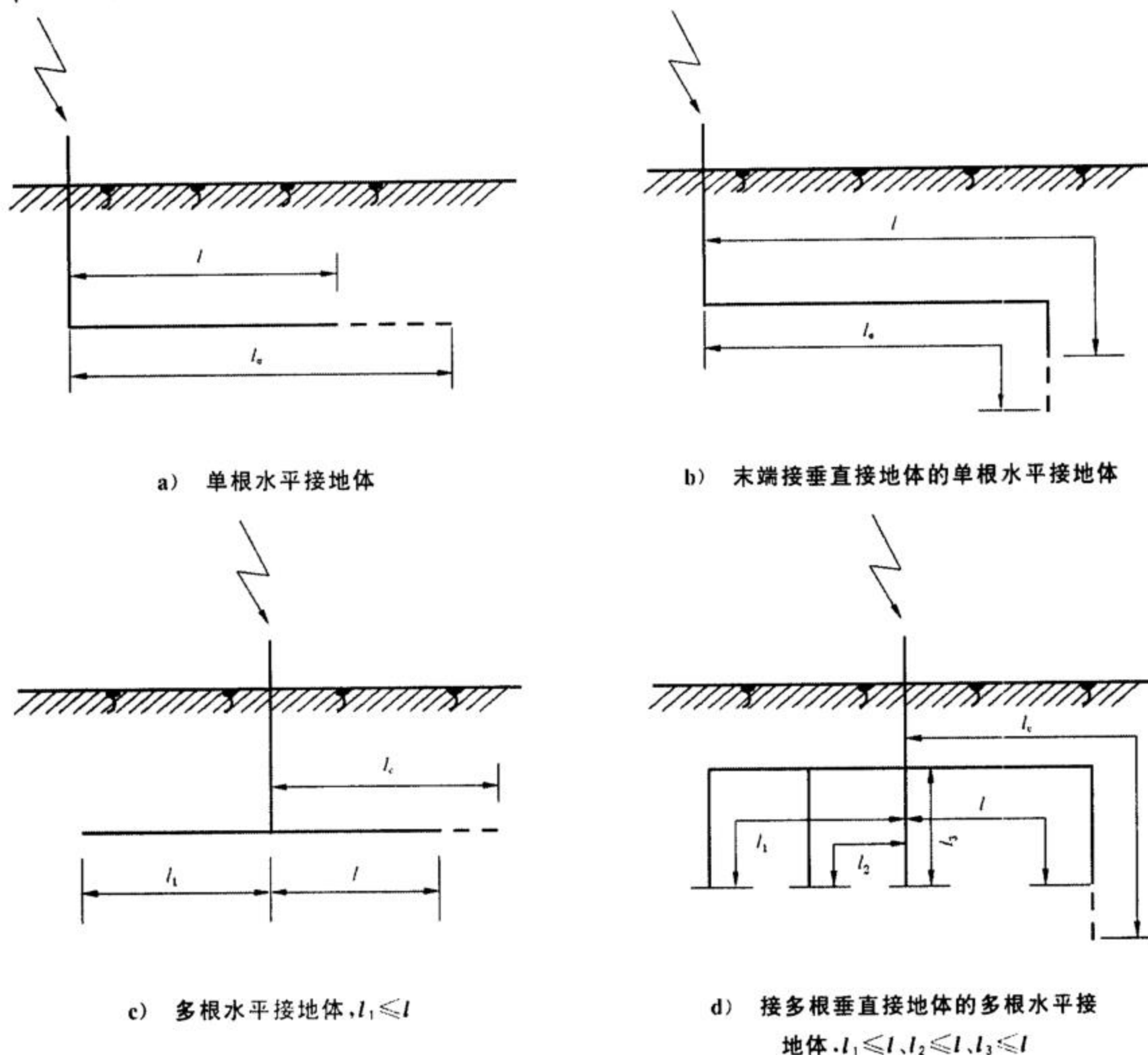
图 H.2 接地体的有效长度
