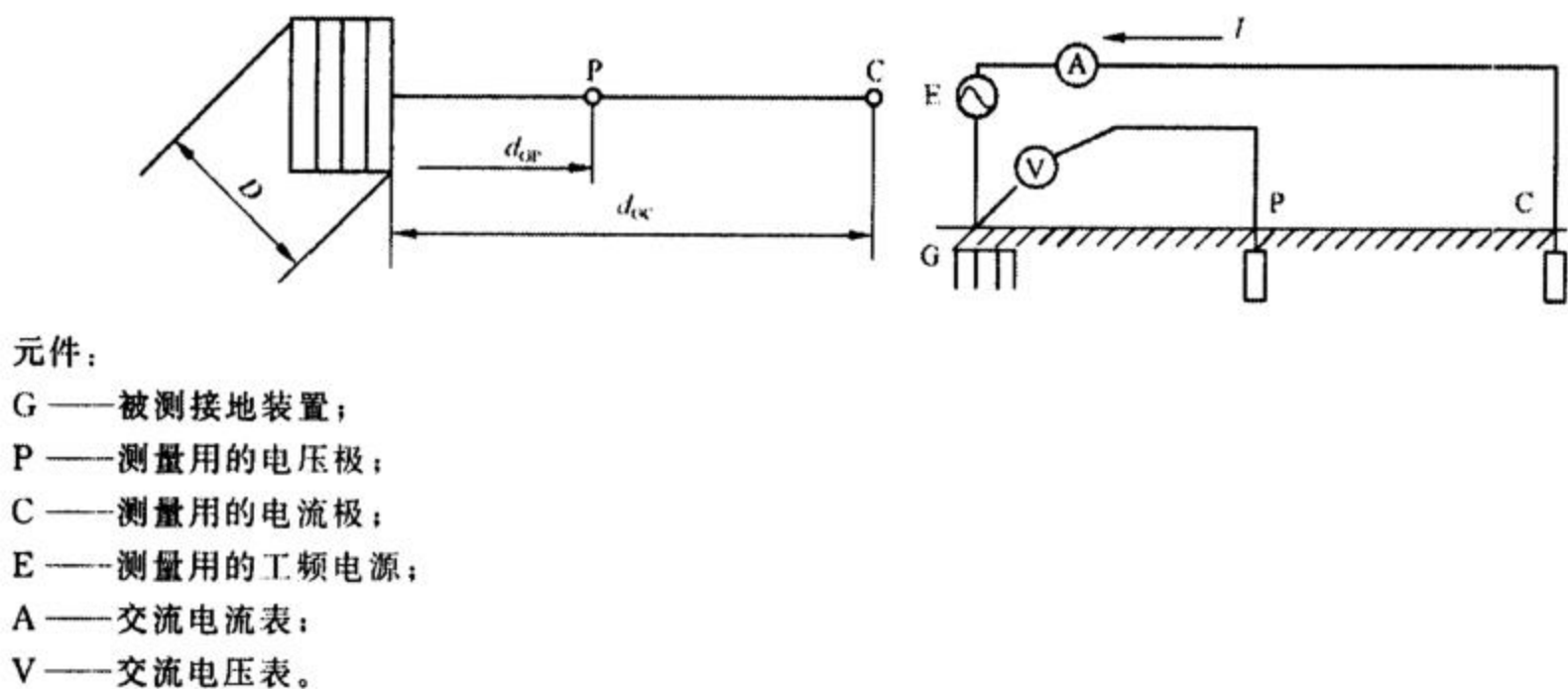
图 F.1 三极法的原理接线图
